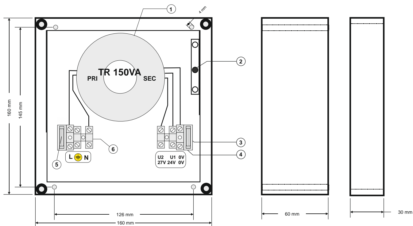
Rys.2. Widok zasilacza.
